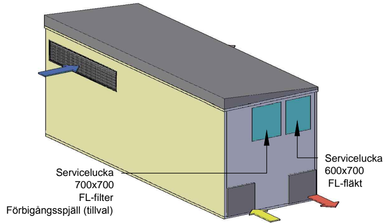
(1:75) 3D Vy bakifrån vänster
