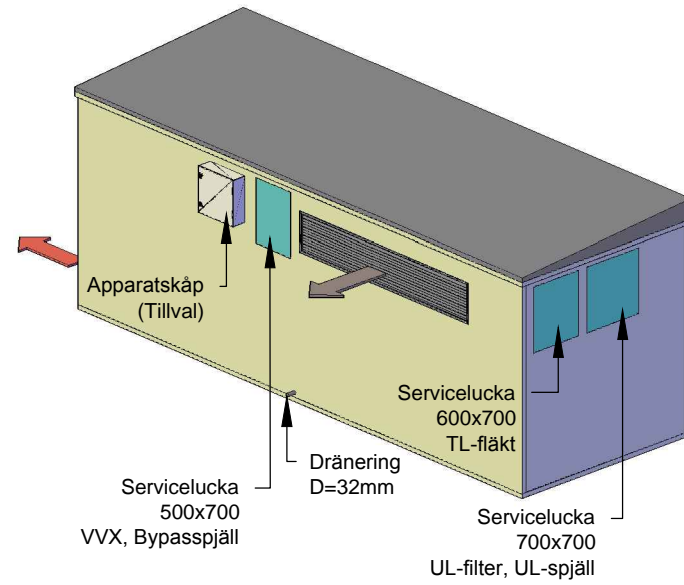
(1:75) 3D Vy framifrån höger
