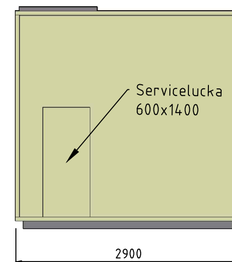
Vänster vy
