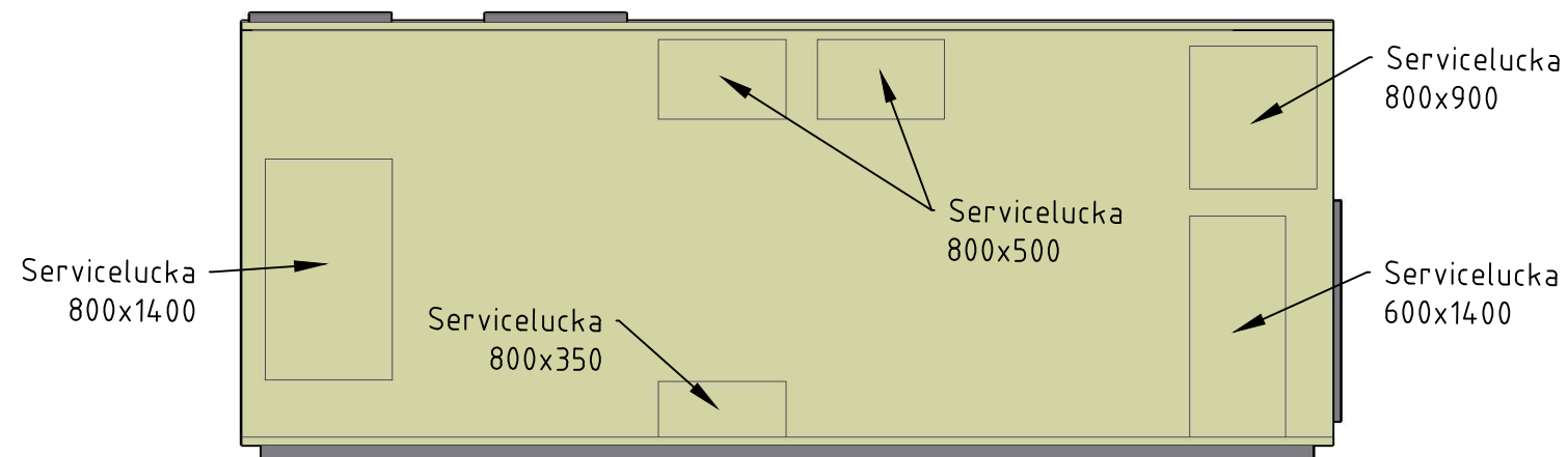
Vy framifrån
